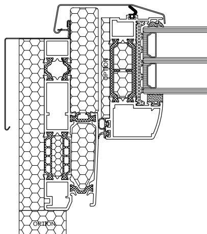
A-A
