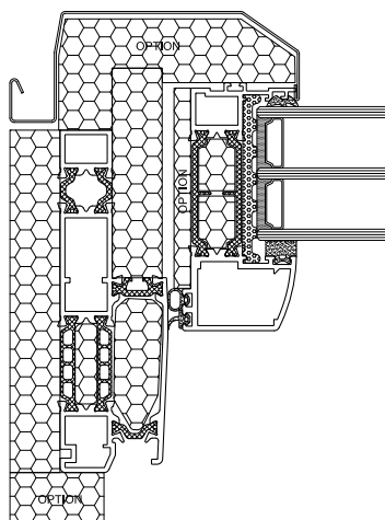
C-C
