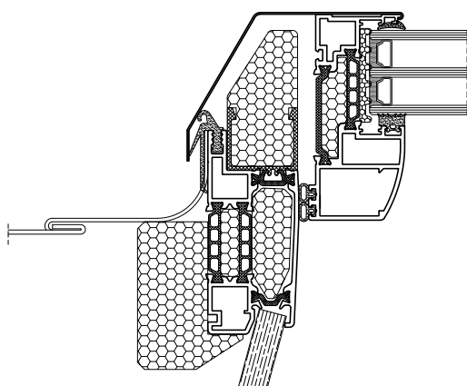
A-A
