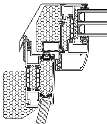
B-B
