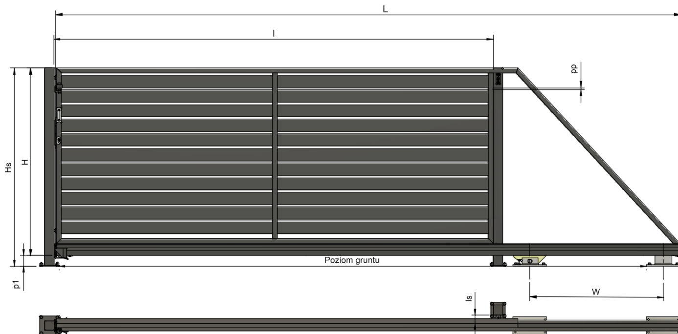
Brama przesuwna ręczna Zegger HORIZONTAL 100 Widok od zewnątrz
