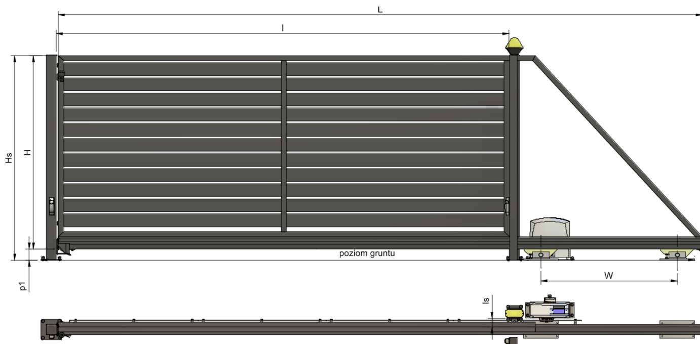
Brama przesuwna automatyczna Zegger HORIZONTAL 100 Widok od zewnątrz
